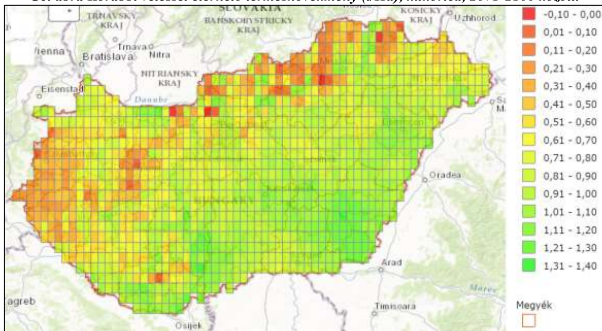
30. ábra Korábbi vetéssel elérhető termésnövekmény (t/Ha), kukorica, 2071-2100 között.
