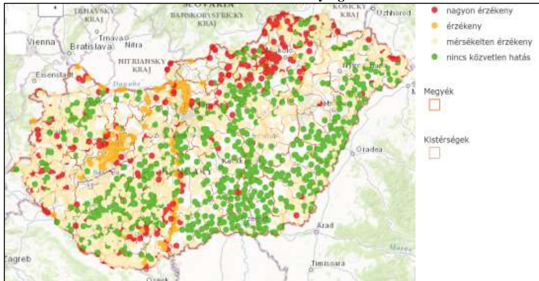
31. ábra Vízbázisok klímaérzékenysége mértéke
