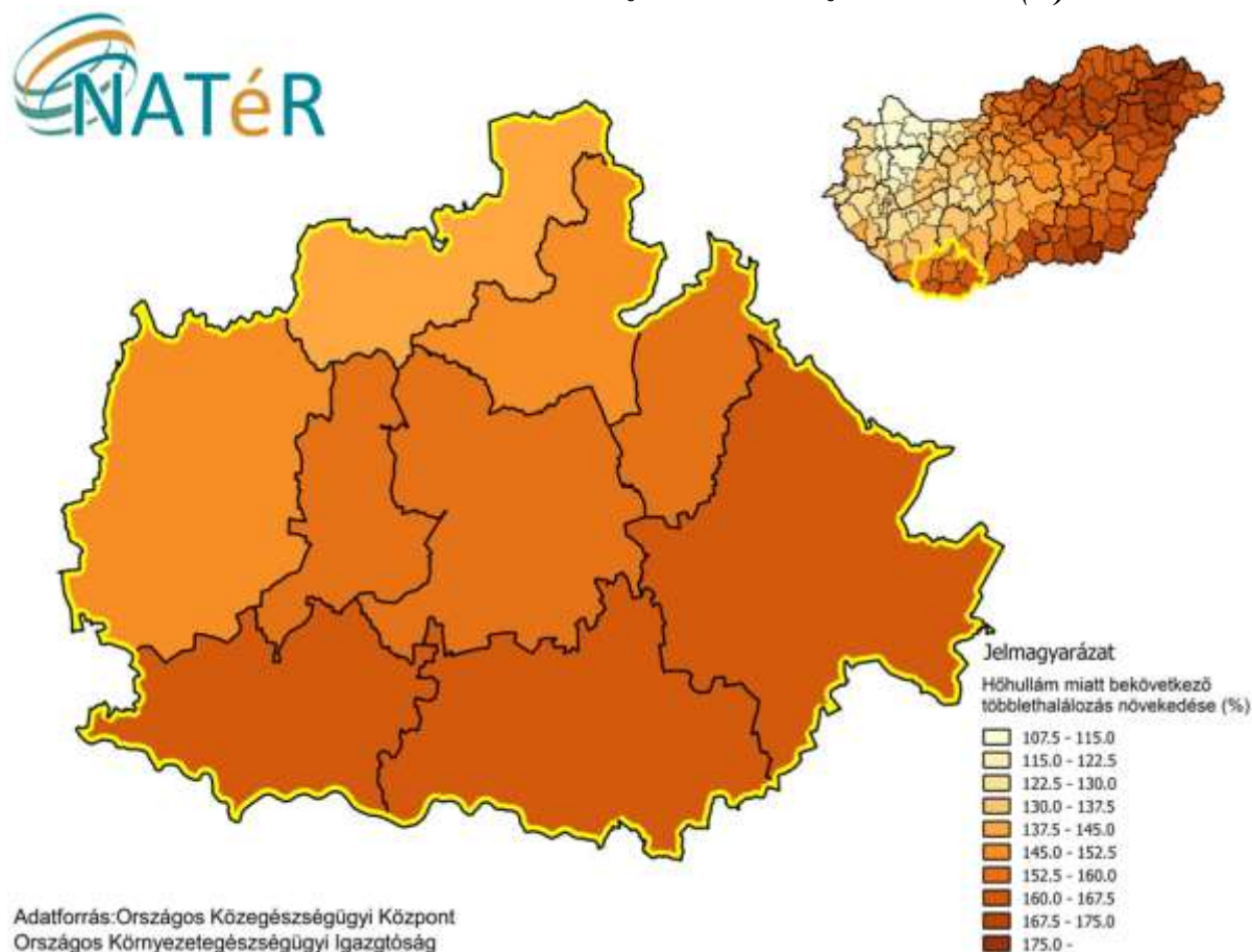
35. ábra Hőhullám miatt bekövetkező többlethalálozás növekedése (%)
