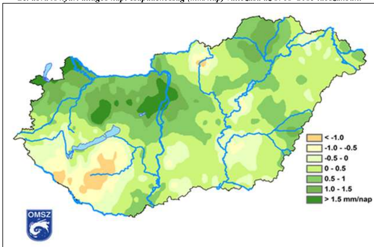
26. ábra A nyári átlagos napi csapadékossg (mm/nap) változása az 1961–2015 időszakban.
